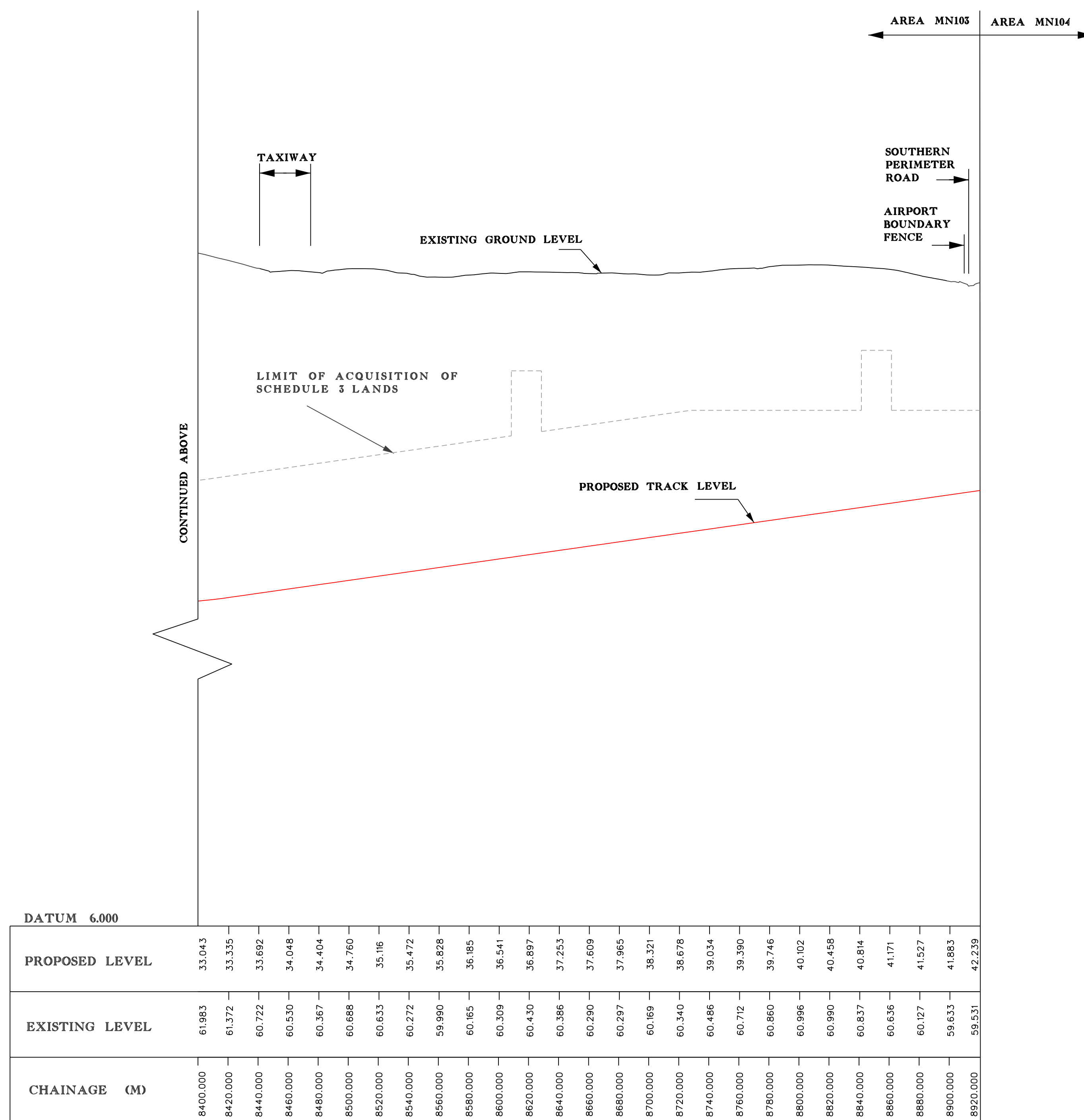
LONGITUDINAL SECTION SCALE: HORZ 1:2000 VERT 1:250
