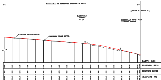
LONGITUDINAL SECTION
